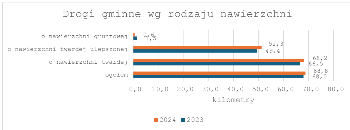
Rysunek 8 Drogi gminne wg rodzaju nawierzchni w gminie Grzegorzew, 2023-2024
